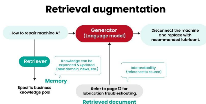
ภาพที่ 2-19 กระบวนการทำงานของ RAG
