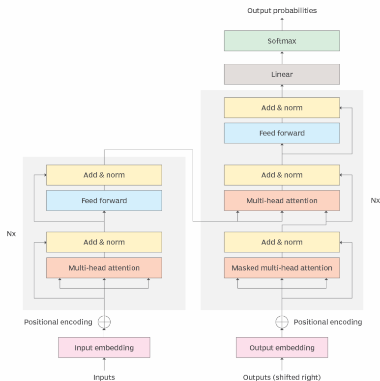
ภาพที่ 2-18 สถาปัตยกรรมโมเดลแบบทรานส์ฟอร์เมอร์
